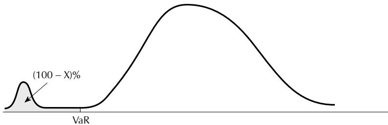
شکل ۲-۱۶: مقدار VaR در این نمودار مشابه نمودار (۱۶-۱) است با این تفاوت که میزان ضرر بالقوه در اینجا بزرگتر است.
